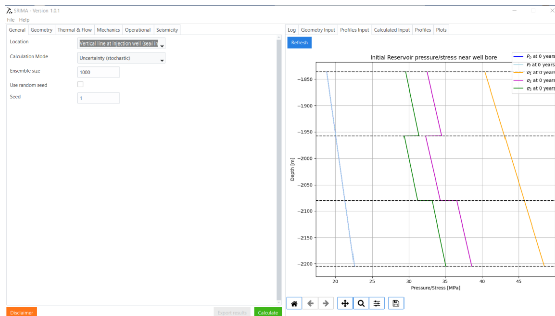
Figuur 3-2: General tabblad van de SRIMA tool. Voor de TAS procedure moet bij locatie “Vertical line at injection well(seal integrity) optie gekozen worden. Voor het stochastische analyse waarbij de onzekerheden in de berekening worden meegenomen moet de calculation mode op “Uncertainty (stochastic) worden gezet.
