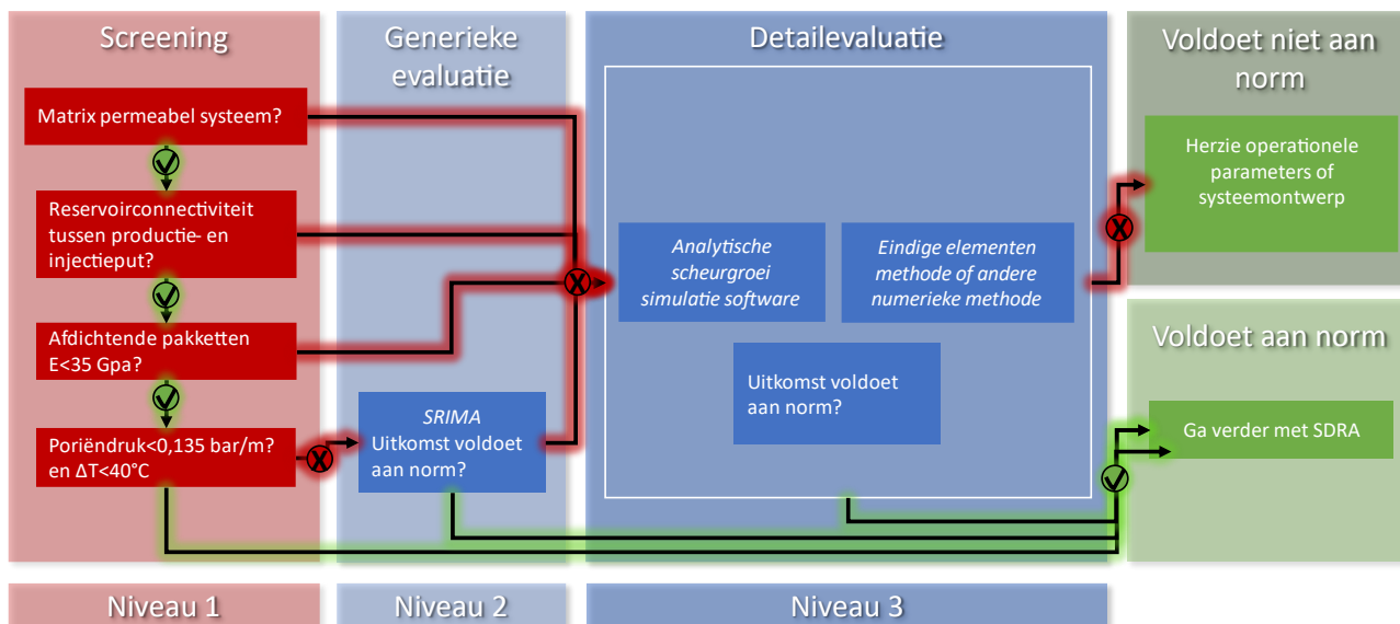
Figuur 3-1: Generiek stappenplan van de TAS-procedure.
