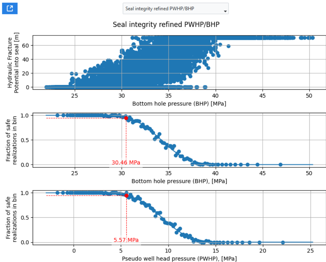
Figuur 3-5: De “Seal/Base integrity refined PWWP/BHP” grafieken van de SRIMA-tool die relevant zijn voor de TAS-procedure. Het debietbereik dat onderliggend is aan deze analyse is niet gelijk aan die van de operationele condities beoogd in het project. De bovenste grafiek geeft de maximale rekscheurhoogte van elke stochastische realisatie. De middelste grafiek geeft per klasse van injectiedruk weer welke fractie van de stochastische berekeningen een maximaal scheurhoogtepotentieel geeft dat aan de norm voldoet. De onderste grafiek lijkt op de middelste, maar dan met klassen voor de pseudo-putkopdruk. Dit is een analyse met 10,000 stochastische realisaties. De fit van de lijn is nu veel beter en daarmee ook definitie van de maximale injectiedruk.
