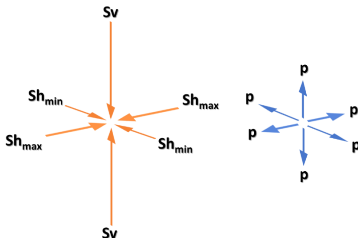
Figuur 1-2: Links) De drie hoofdcomponenten van ondergrondse spanning op een willekeurig referentiepunt in de ondergrond: De verticale spanning, S_v , de minimale horizontale spanning, Sh_{min} en de maximale horizontale spanning Sh_{max} . De lengte van de pijlen geven het onderlinge verschil aan in spanningsgrootte zoals deze in de Nederlandse ondergrond heerst. Deze specifieke situatie wordt door geologen omschreven als een normaal spanningsregime. Rechts) De poriëndruk, p , op een willekeurig referentiepunt in de ondergrond wordt in een goed doorlatend gesteentepakket bepaald door de bovenliggende waterkolom. De grootte van deze spanning is gelijk in alle richtingen.
