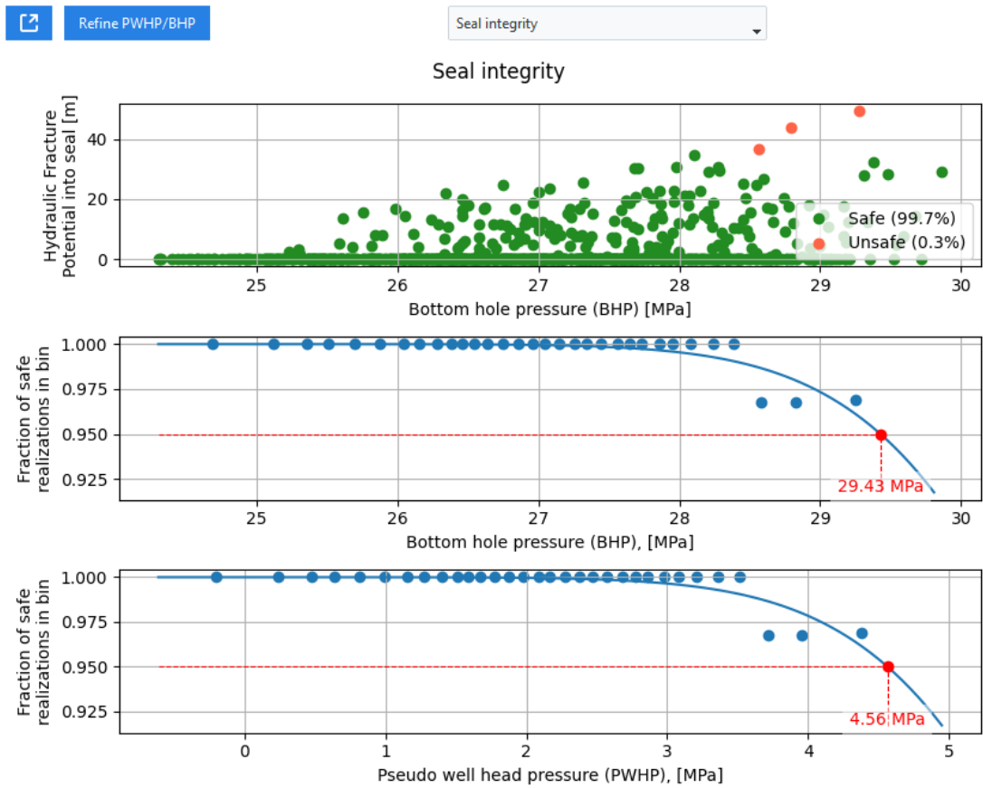
Figuur 3-4: De eerste orde benadering “seal failure plots” grafieken van de SRIMA-tool die relevant zijn voor de TAS-procedure. De bovenste grafiek geeft de maximale rekscheurhoogte van elke stochastische realisatie. De rode punten voldoen niet aan de norm de groene wel. De middelste grafiek geeft per klasse van putvoetdruk (BHP) weer welk deel van de stochastische berekeningen het maximale scheurhoogtepotentieel aan de norm voldoet. De onderste grafiek lijkt op de middelste, maar dan met klassen voor de pseudo-putkopdruk. Dit is een analyse met 1000 stochastische realisaties. Zoals te zien is zijn er in het hoge drukk bereik (gerelateerd aan de opgegeven debieten) te weinig punten om de curve goed te fitten. Nadere analyse kan worden uitgevoerd door op de “Refine PWHP/BHP” (psuedo well head pressure/Bottom hole pressure) knop te drukken.
